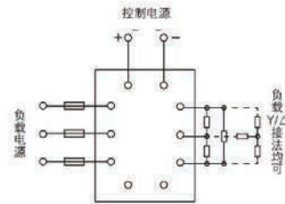
应用电路接线图
