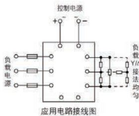
应用电路接线图
