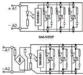
典型内部电路图
